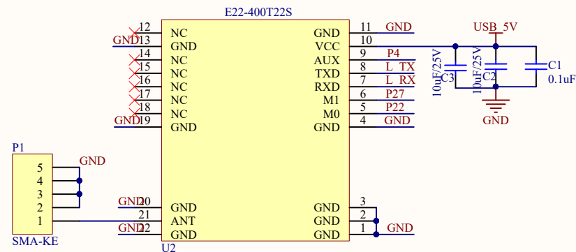
LoRa Module
